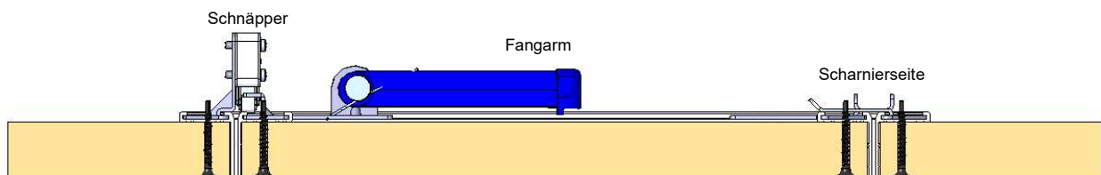
Skizze: Einbaubeispiel mit einer bauseits verschraubten 25mm Einlage
