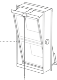
Lüftungsflügel für 2 Glasbausteine
